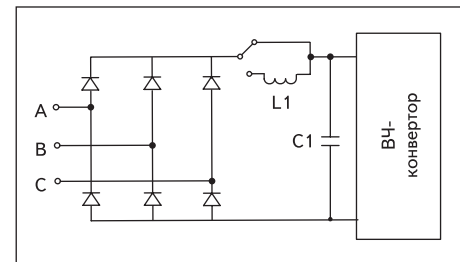
Рис. 5. Трехфазный мост с фильтром C и LC
