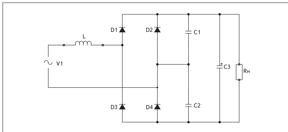
Рис. 1. Принципиальная схема корректора коэффициента мощности
