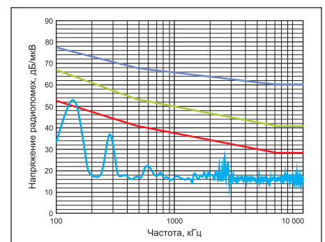
Рис. 4. Входная спектрограмма для модуля с фильтром на входе
