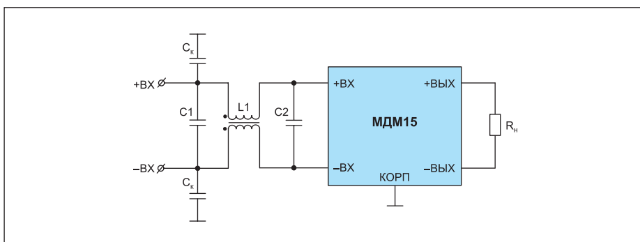
Рис. 3. Модуль МДМ15 с фильтром на входе. C1, C2 = 33 мкФ \times 100 В, C_x = 0,47 мкФ \times 100 В, L1 — дроссель ДФ15-2Р/3
